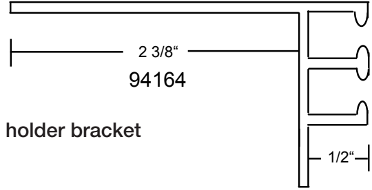
Long Flange
